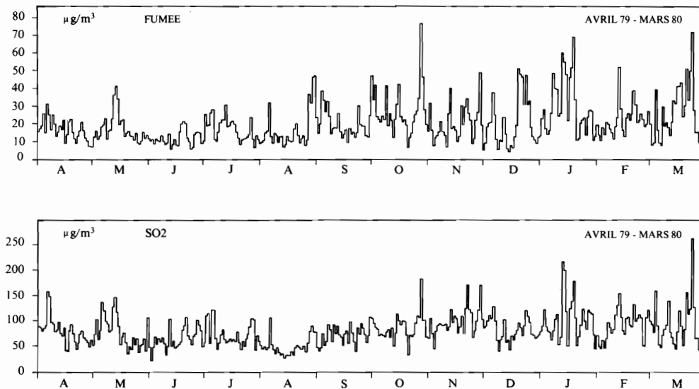
Pollution moyenne à Anvers
